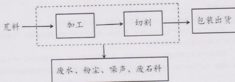
图 2-3 项目生产流程及产污节点图
