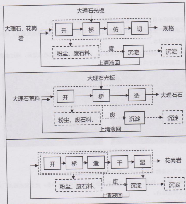
主要工艺流程及产物环节（附处理工艺流程图，标出产污节点）
