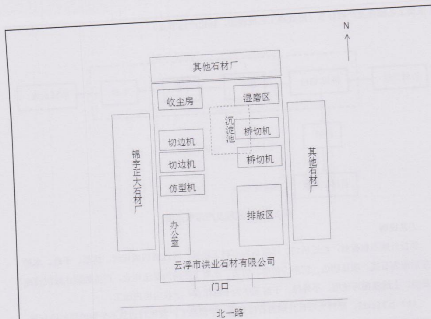
图2-1项目平面布置图
