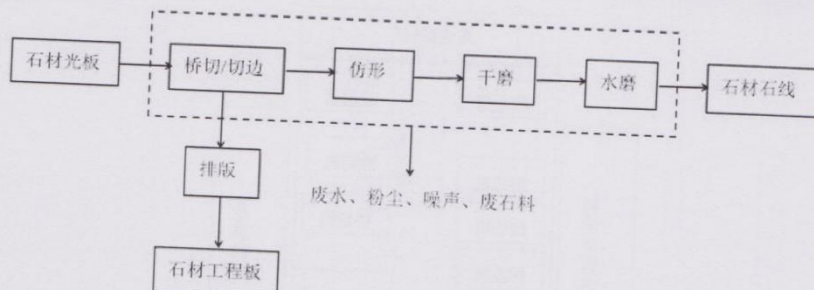
图 2-2 生产流程及产污节点图
