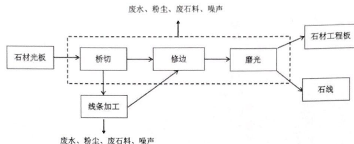
图 2-3 项目生产流程及产污节点图
