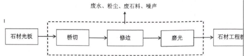
图 2-3 项目生产流程及产污节点图
