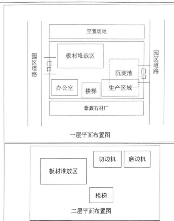
图2-1 项目平面布置图
