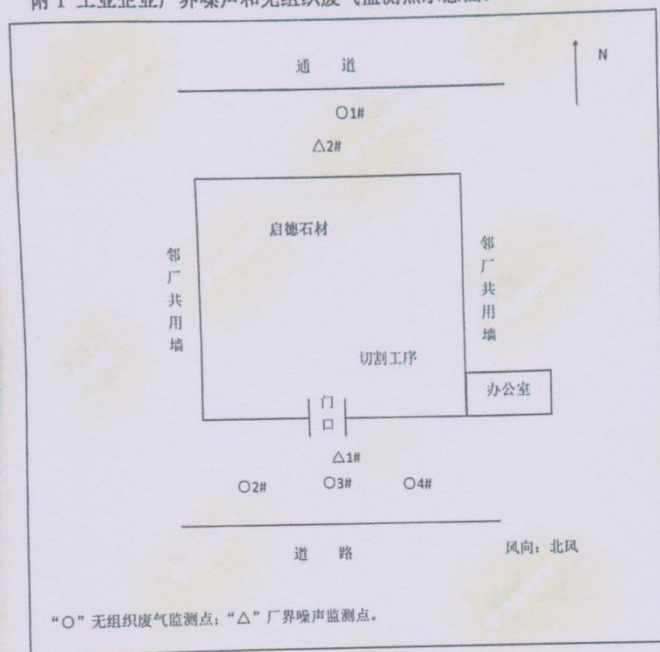
附1 工业企业厂界噪声和无组织废气监测点示意图:
