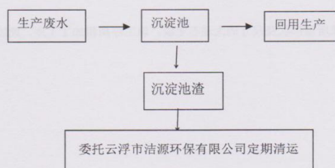
图2-1废水流向示意图
