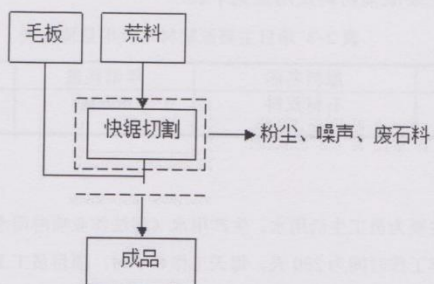
图 2-3 项目生产流程及产污节点图
