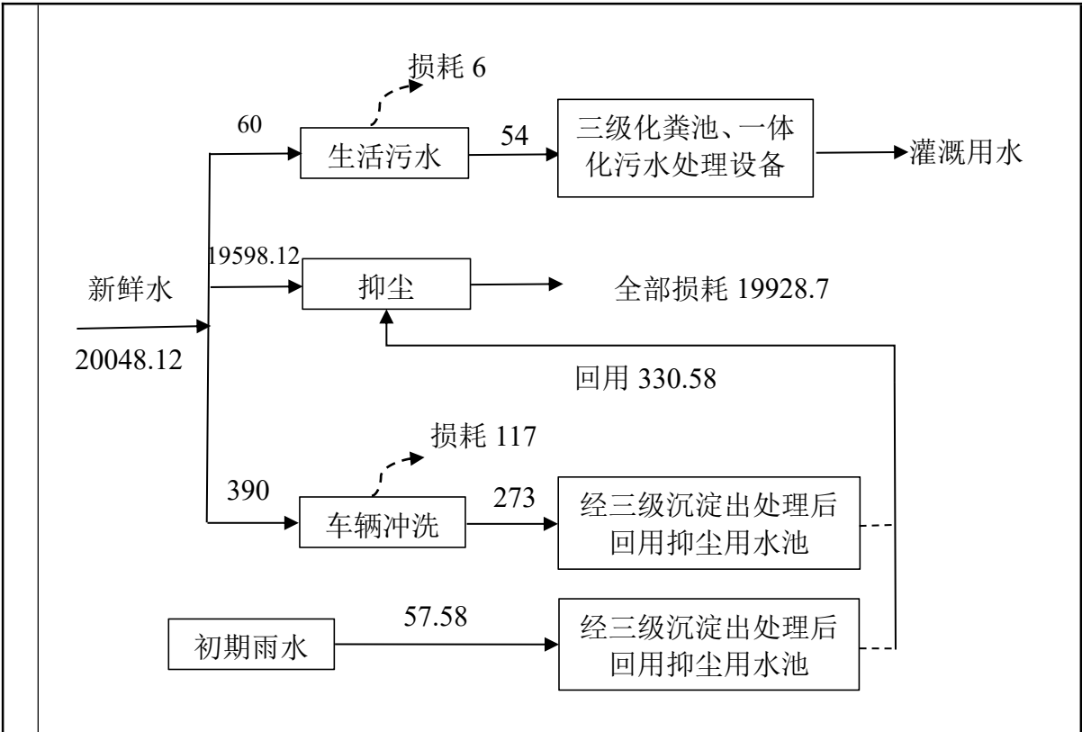
图 4-2 项目水平衡图（m³/a）
