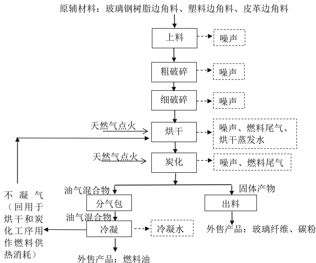
图 2-3 项目工艺流程图
